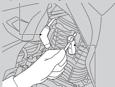
Llave de bujías
